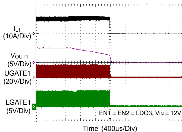
VOUT1 UVP
